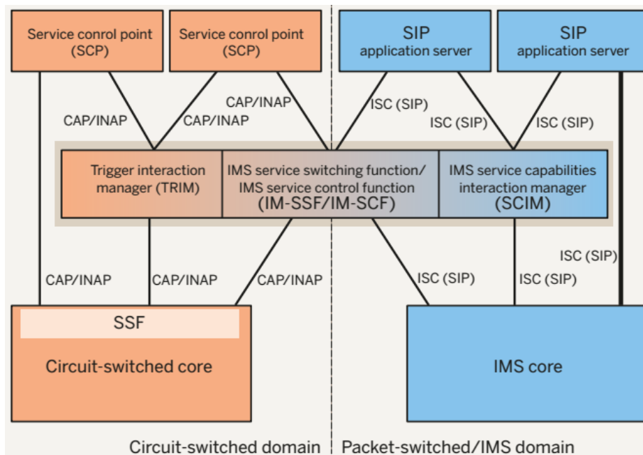
Figura 1: Arquitectura de NGIN.
