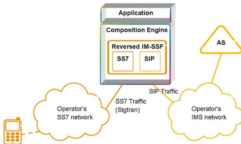
Figura 4: ECE con función de IM-SSF invertido.
