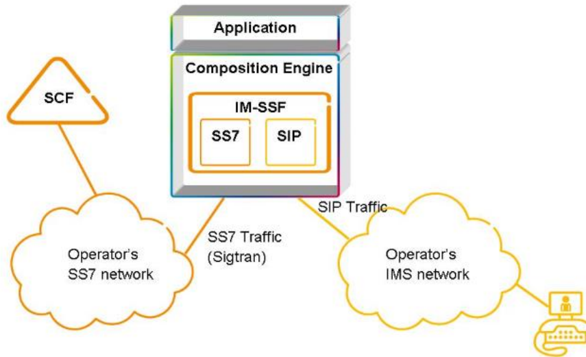
Figura 2: ECE con función de IM-SSF.
