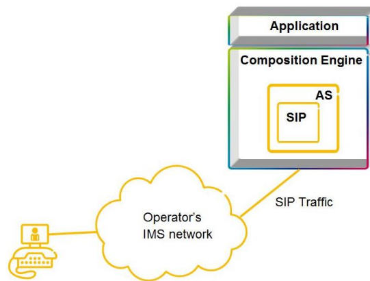
Figura 5: ECE con función de SIP-AS.
