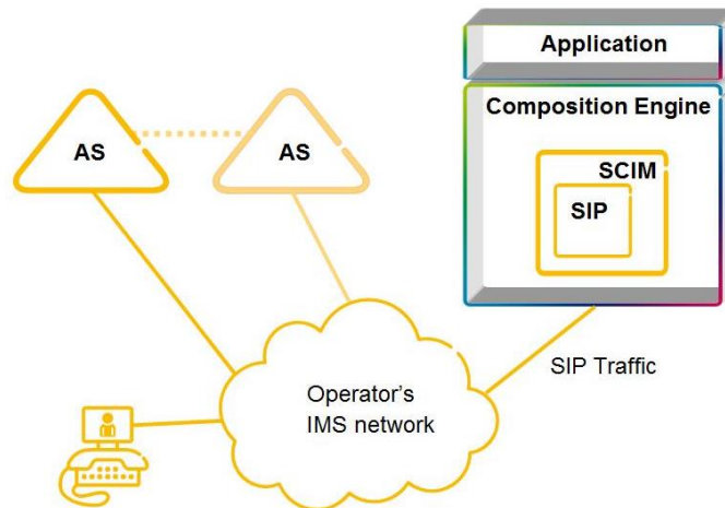
Figura 6: ECE con función de SCIM.
