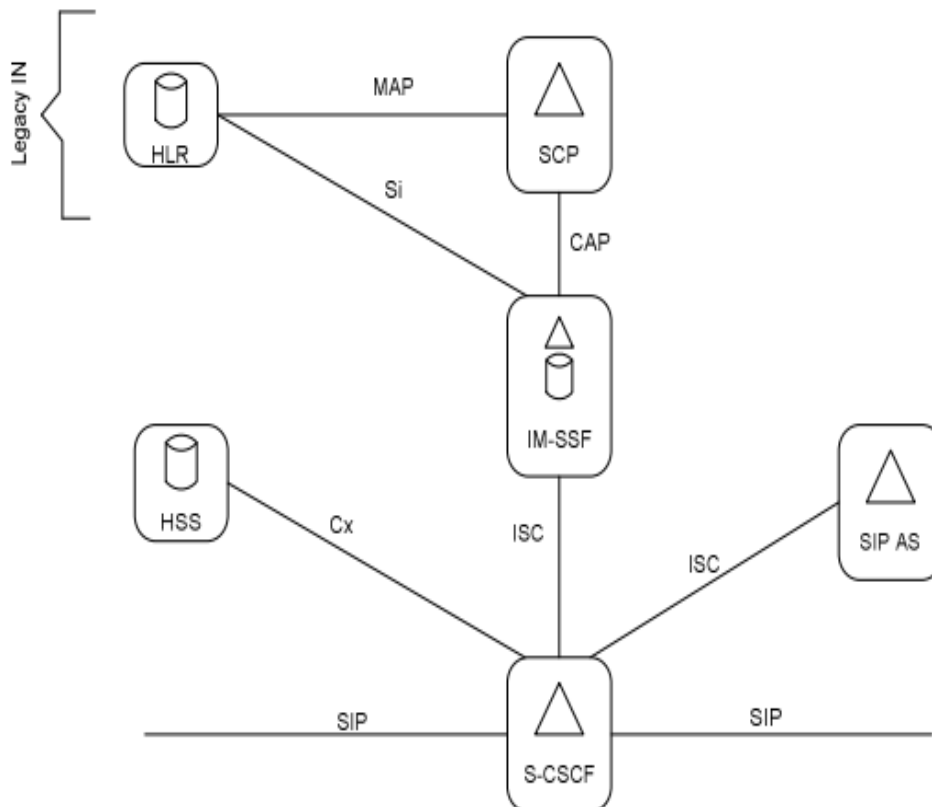
Figura 3: IM-SSF invertido para la integración de las redes legadas con IMS.
