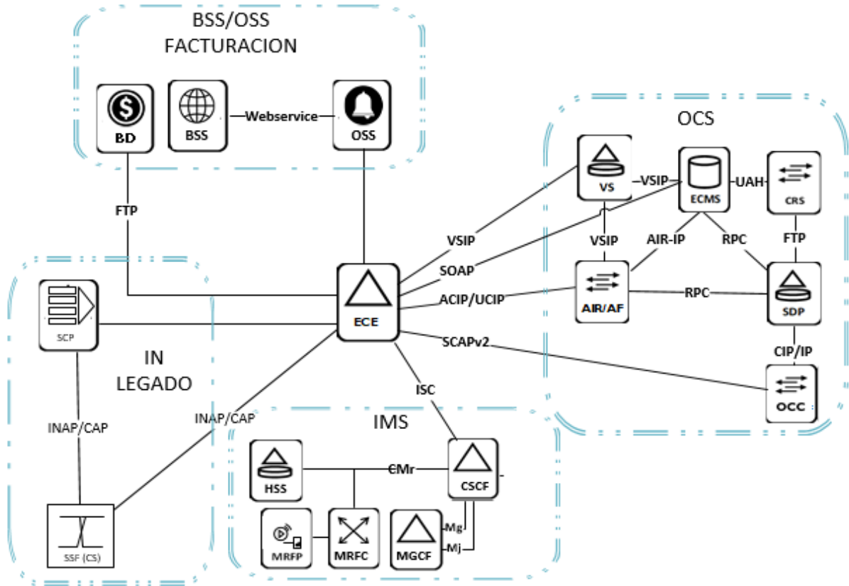
Figura 8: ECE integrado con otras plataformas.
